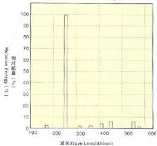
● 石英灯 Ozone Lamp
