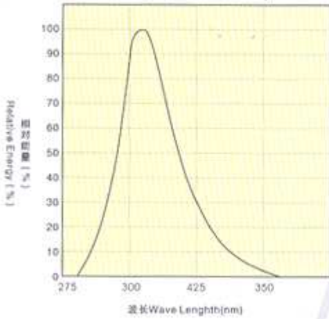
● UV-B灯 UV-B Lamp
